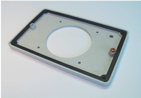
bearbeiteter Gussdeckel mit Flachdichtung
